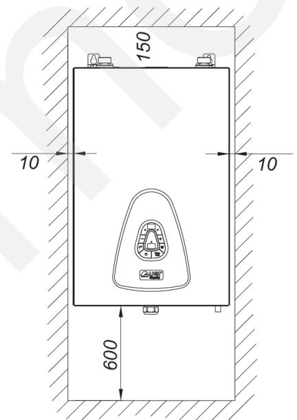
Σχήμα 5: Αποστάσεις από σταθερά σημεία..
