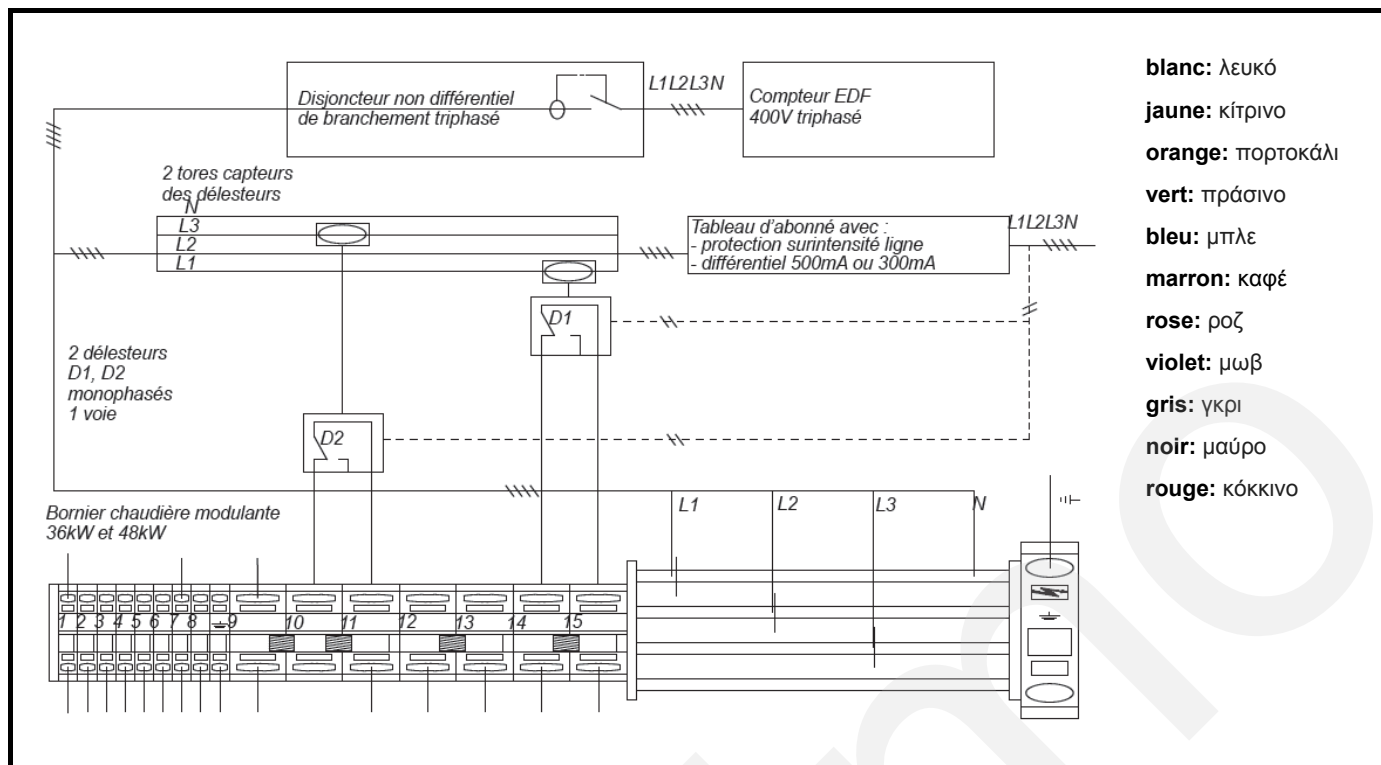
Σχήμα 9: Ηλεκτρική σύνδεση των ρελέ των ηλεκτρικών στοιχείων Applimo 36MA - 48MA .
