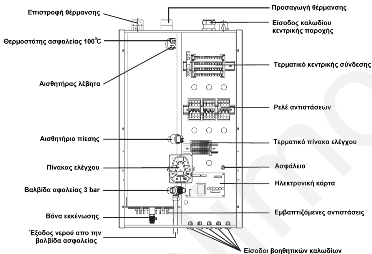
Σχήμα 1 : Λέβητας Applimo 36kW-72kW.
