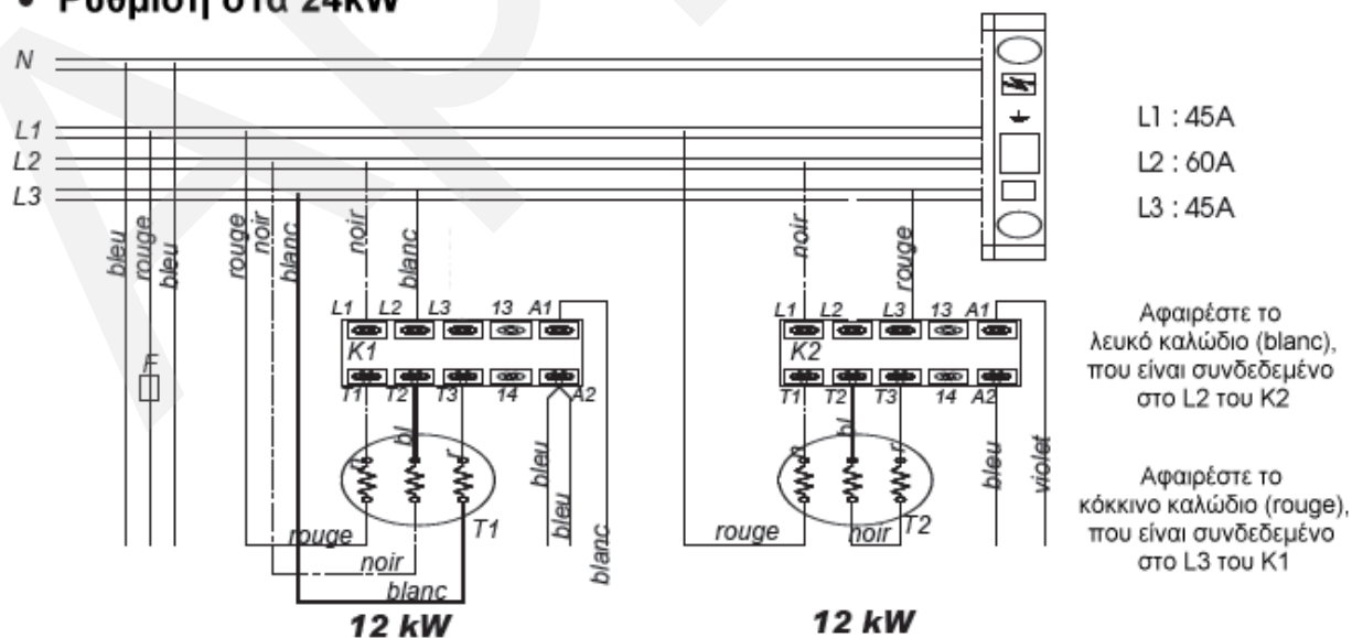
Σχήμα 17: Μεταβολή της ισχύος του λέβητα Gialix 36MA με αφαίρεση καλωδίων.
