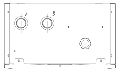
Σχήμα 6 : Άνω όψη λέβητα
