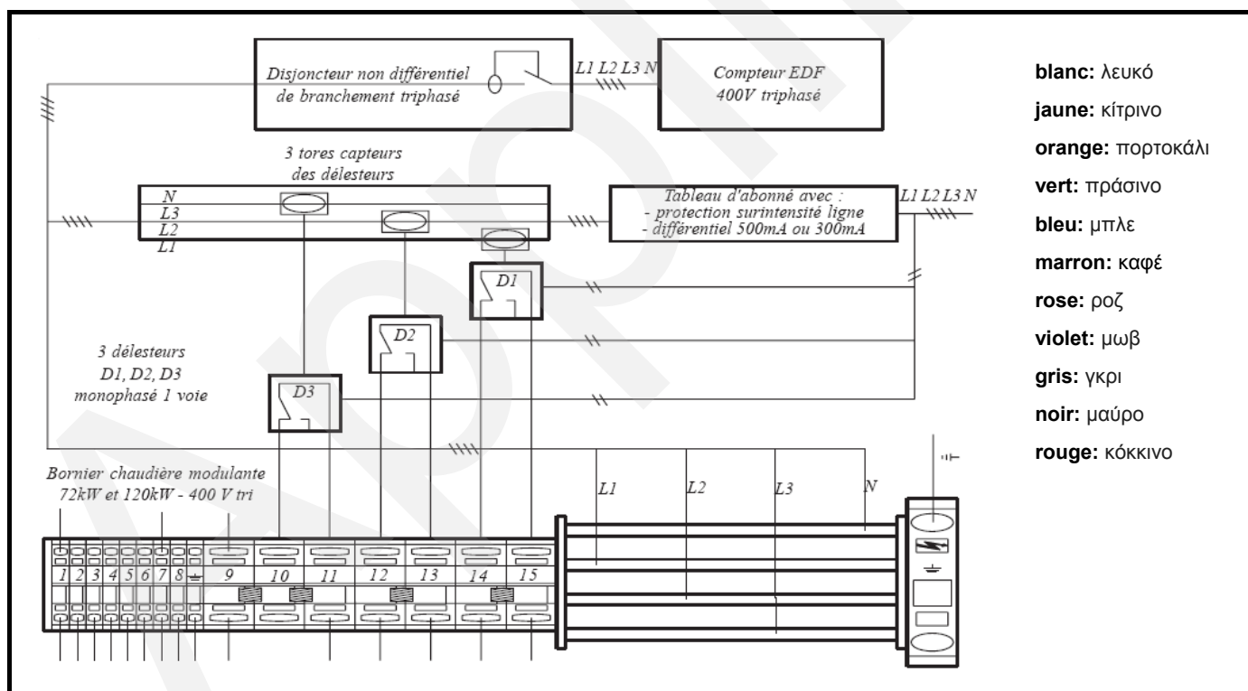
Σχήμα 10: Ηλεκτρική σύνδεση των ρελέ των ηλεκτρικών στοιχείων Applimo 72MA .
