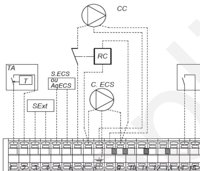
Σχήμα 16: Ηλεκτρική συνδεσμολογία για εγκατάσταση με δυο κυκλοφορητές.
