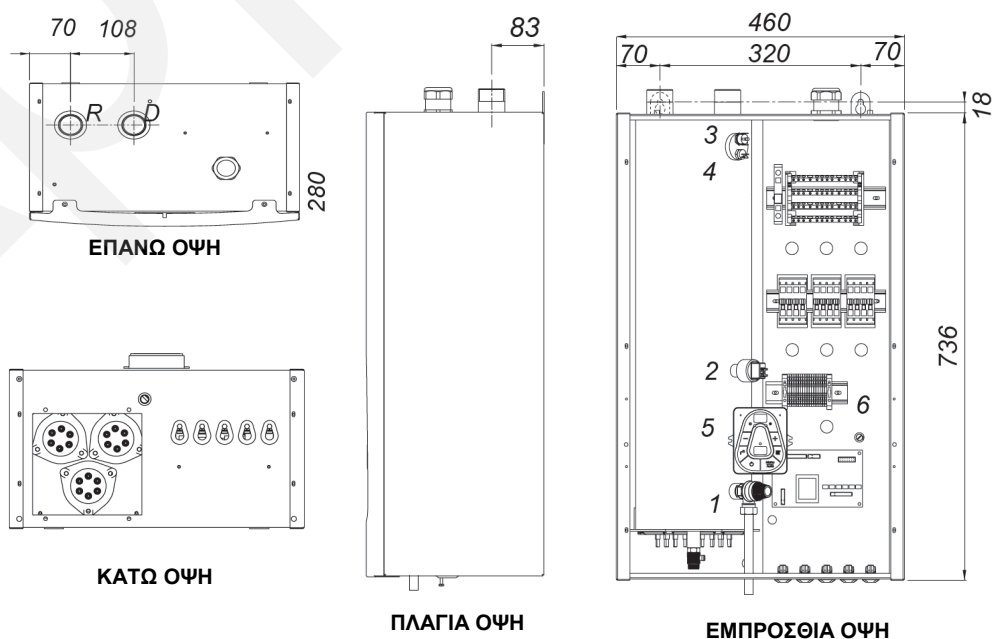
Σχήμα 2 : Βασικές διαστάσεις λέβητα Applimo 36kW-72kW.
