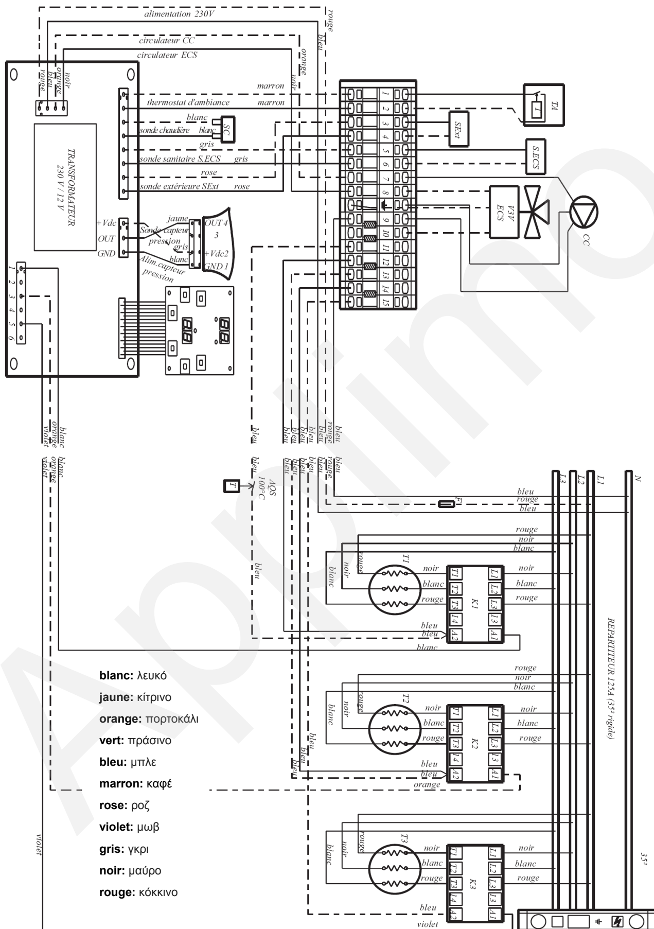
Σχήμα 14: Ηλεκτρική συνδεσμολογία Applimo 72MA
