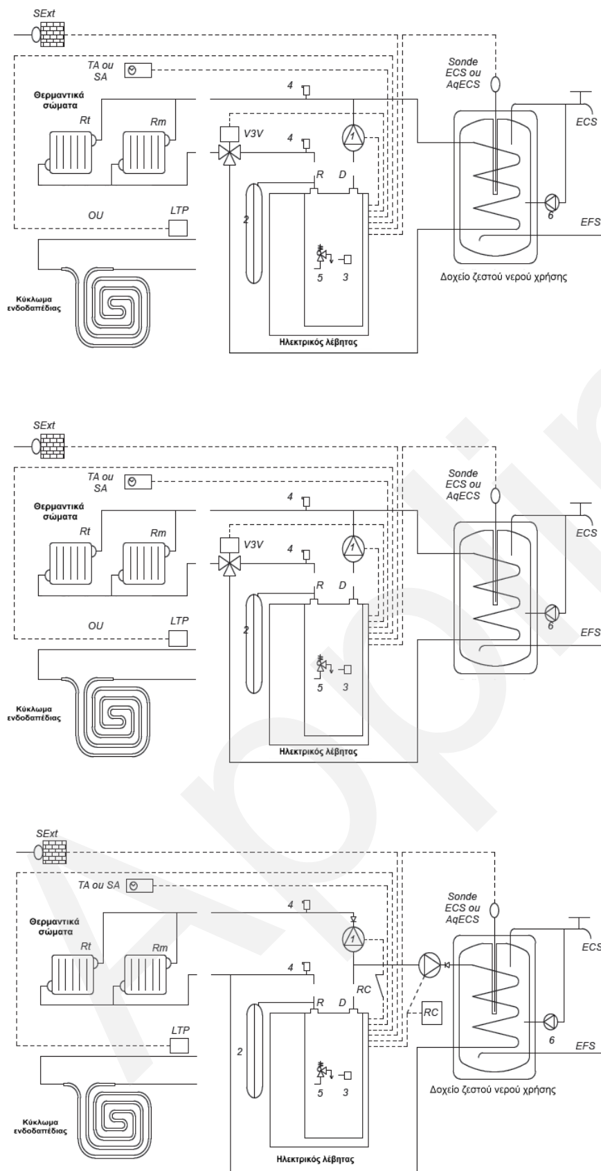
Σχήμα 7: Σύνδεση ηλεκτρικού λέβητα Applimo MA με σύστημα θέρμανσης.
