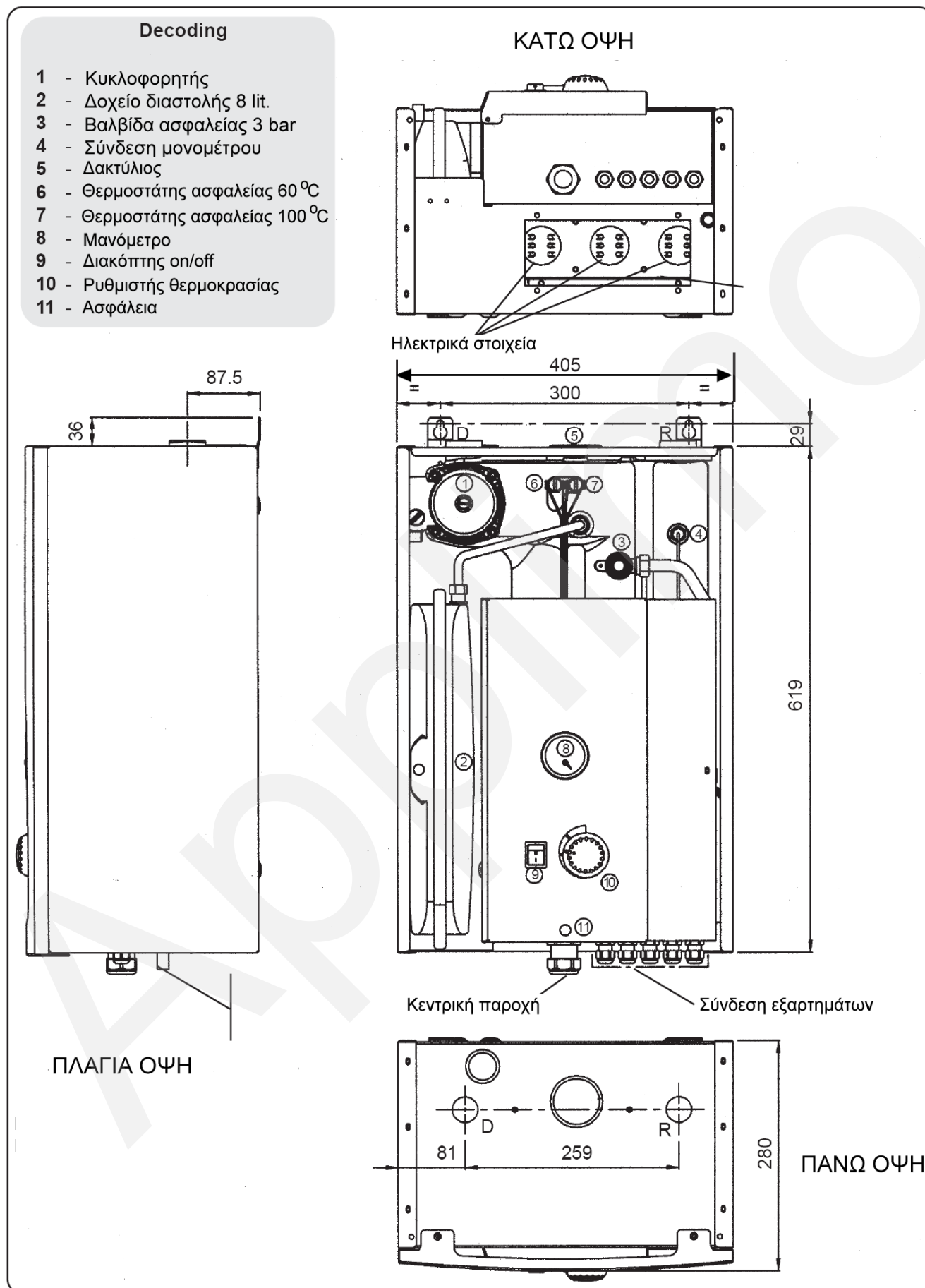
Σχήμα 3 : Διαστάσεις - Υδραυλικές συνδέσεις
