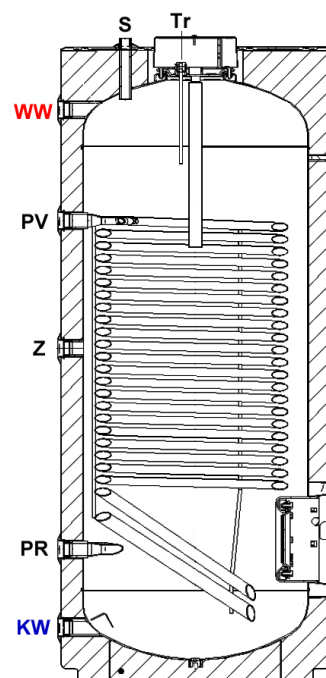
Δυνατότητα προσθήκης φλάντζας με ηλεκτρική αντίσταση ή εναλλάκτη.
