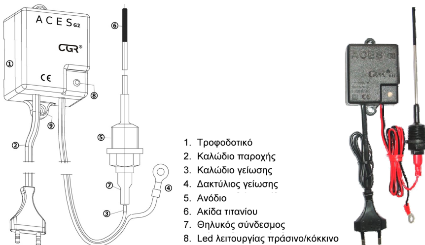
Σχήμα 1: Σύστημα ACES G2 για μπόιλερ έως και 1.000 lit. με ένα ανόδιο τιτανίου.
