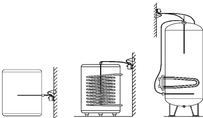
Σχήμα 3: Παραδείγματα τοποθέτησης ανοδίων
