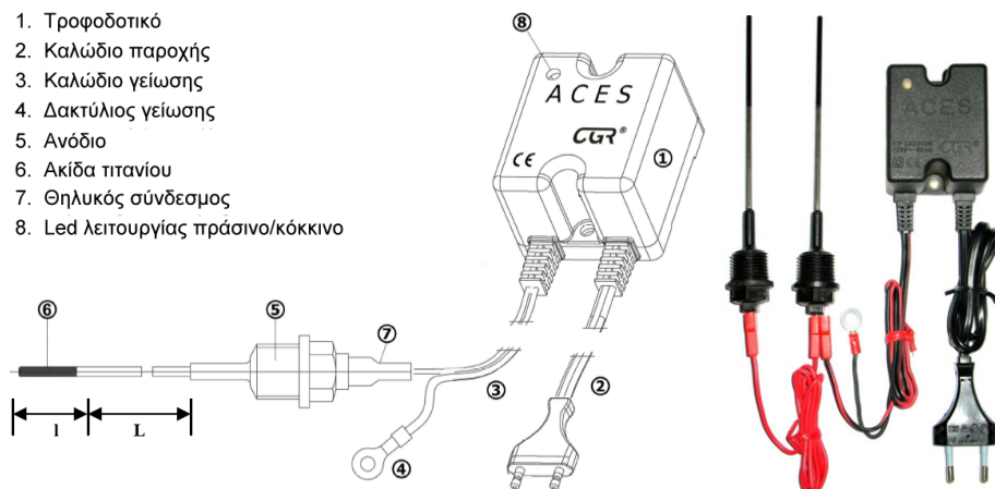
Σχήμα 2: Σύστημα ACES H για μπόιλερ από 1.000 έως και 5.000 lit. με 1 ή δυο ανόδια τιτανίου.
